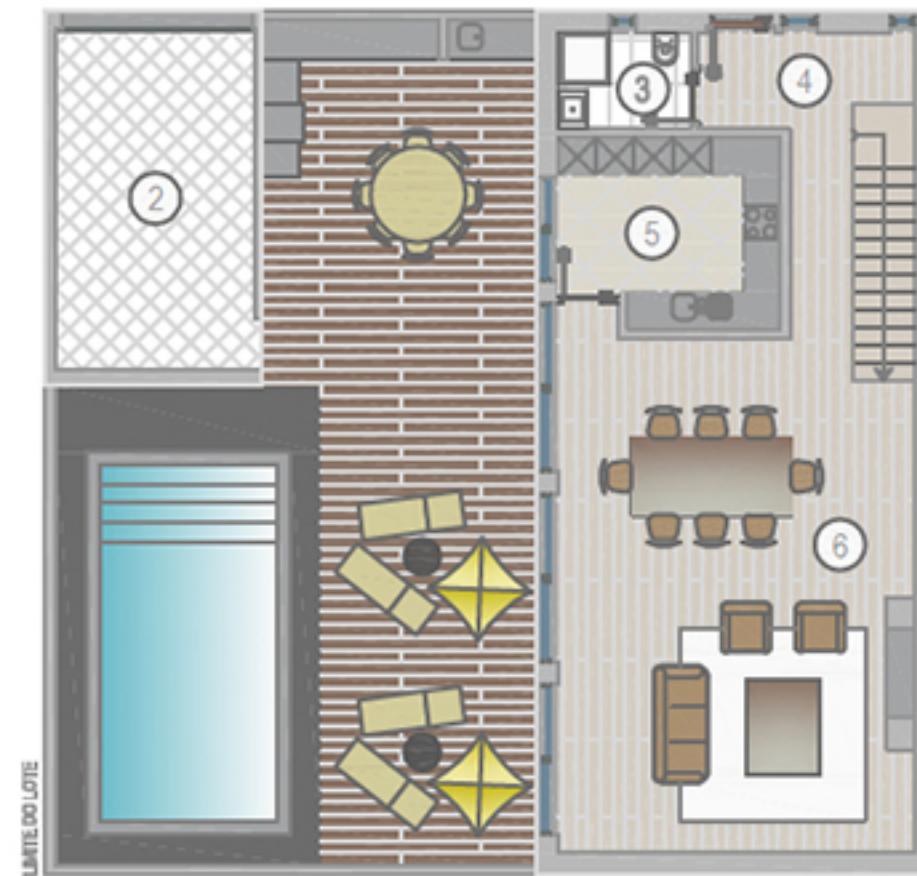
R/ CHÃO ÁREA BRUTA=85,95 m 2 GARAGEM=20,12 m 2
